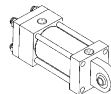
Tipo SBb Articulação traseira macho com Rótula Página 28
