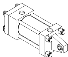
Tipo SB Articulação traseira macho com rótula Página 26
