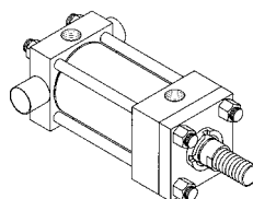
Tipo SBa Articulação traseira macho com rótula (ISO 6982 e CETOP RP88H) Página 27
