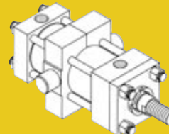
Tipo DD Munhão fixo intermediário (NFFA Tipo MT4) Página 24
