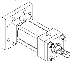
Tipo HB Flange quadrado traseiro (NFFA Tipo MF6) Página 20
