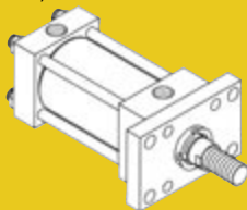
Tipo J Flange retangular dianteiro (NFFA Tipo MF1) Página 18
