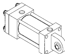
Tipo SBa Articulação traseira macho com rótula (ISO 6982 e CETOP RP88H) Página 27
